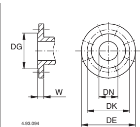
Фланцы PN 10, EN 1092-2EN 1092-2
